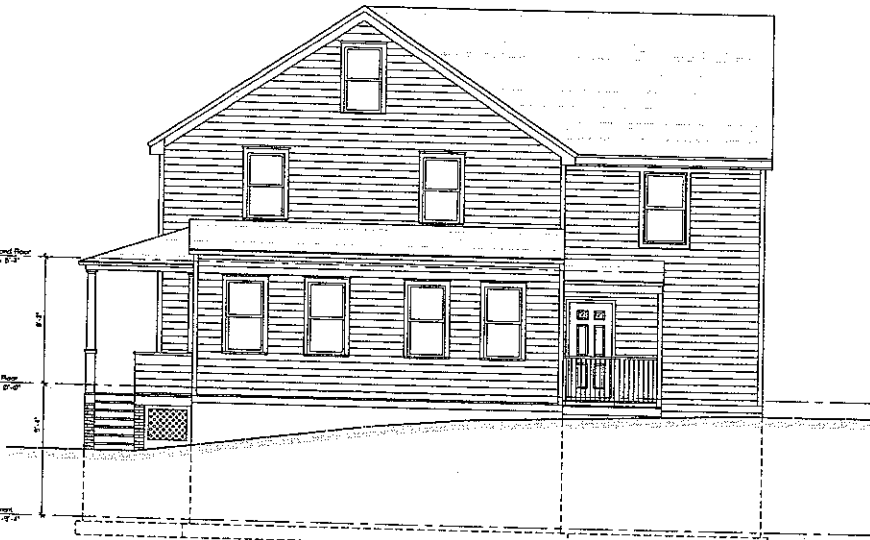
2 SIDE ELEVATION SCALE: 1/4" = 1'-0"
