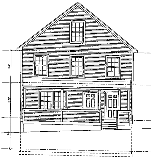
1 FRONT ELEVATION SCALE: 1/8" = 1'-0"
