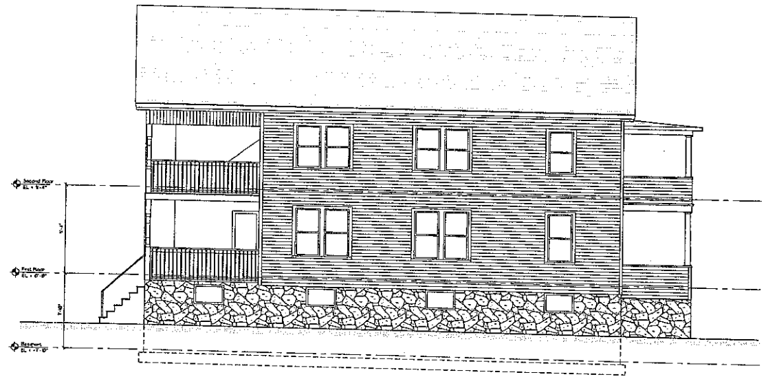
② LEFT ELEVATION SCALE: 1/4" = 1'-0"
