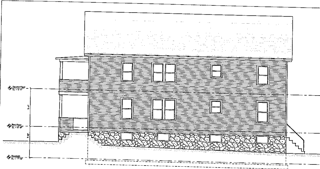
④ RIGHT ELEVATION SCALE: 1/4" = 1'-0"
