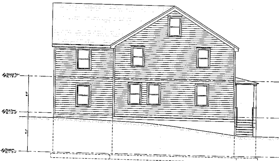
4 SIDE ELEVATION SCALE: 1/4" = 1'-0"
