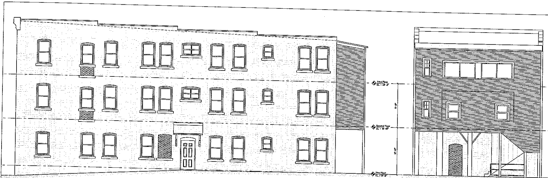
4 RIGHT ELEVATION SCALE: 1/4" = 1'-0"
