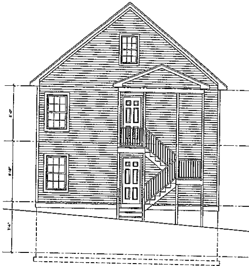
3 REAR ELEVATION SCALE: 1/8" = 1'-0"
