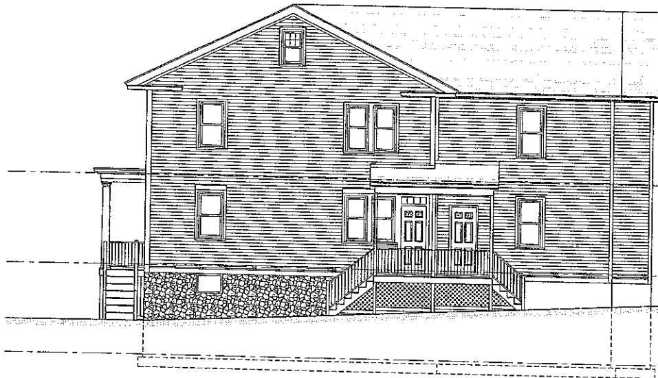
④ RIGHT ELEVATION SCALE: 1/4" = 1'-0"
